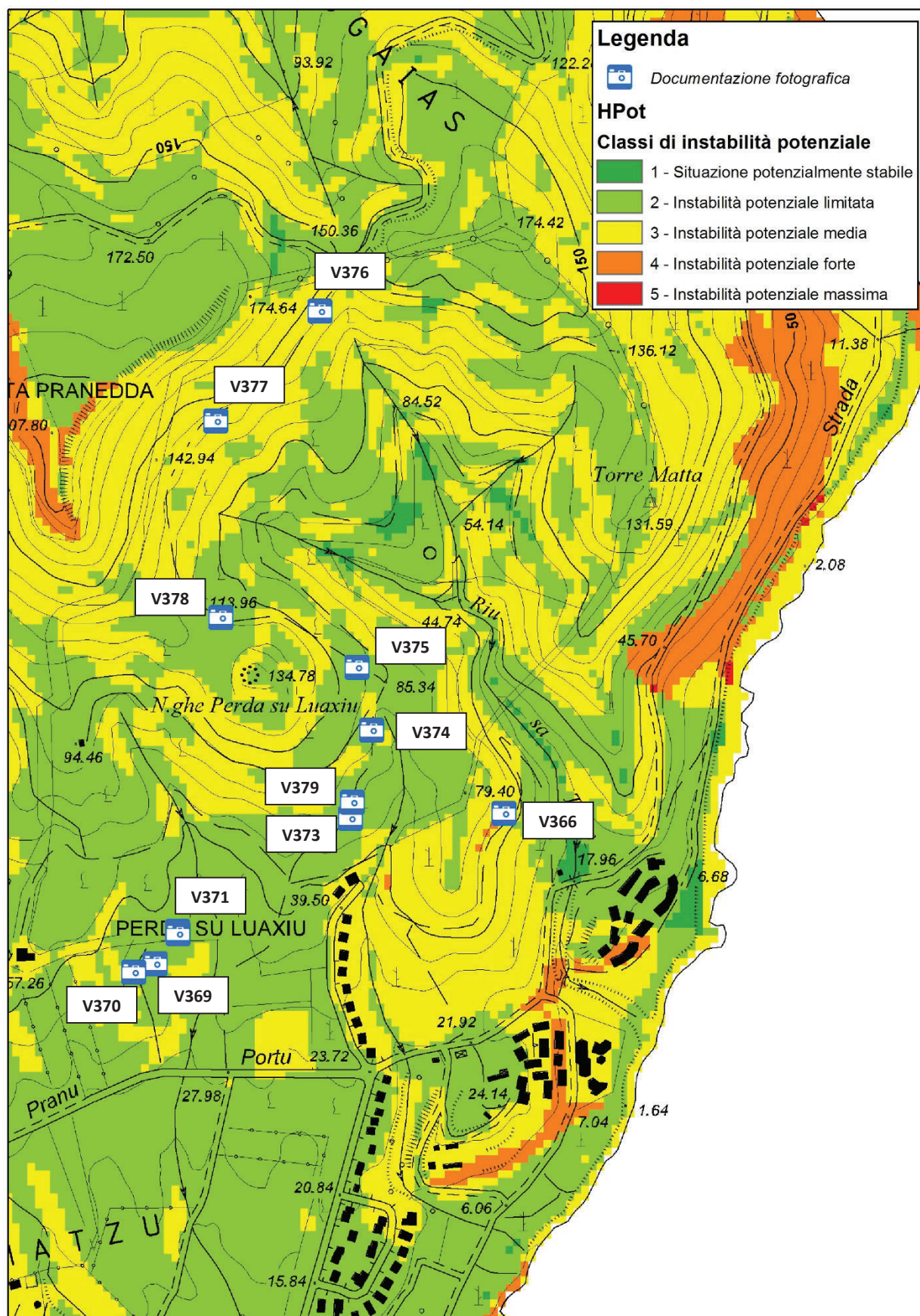
Figura 22 – Carta di instabilità potenziale per l'area a Nord di Porto Corallo
