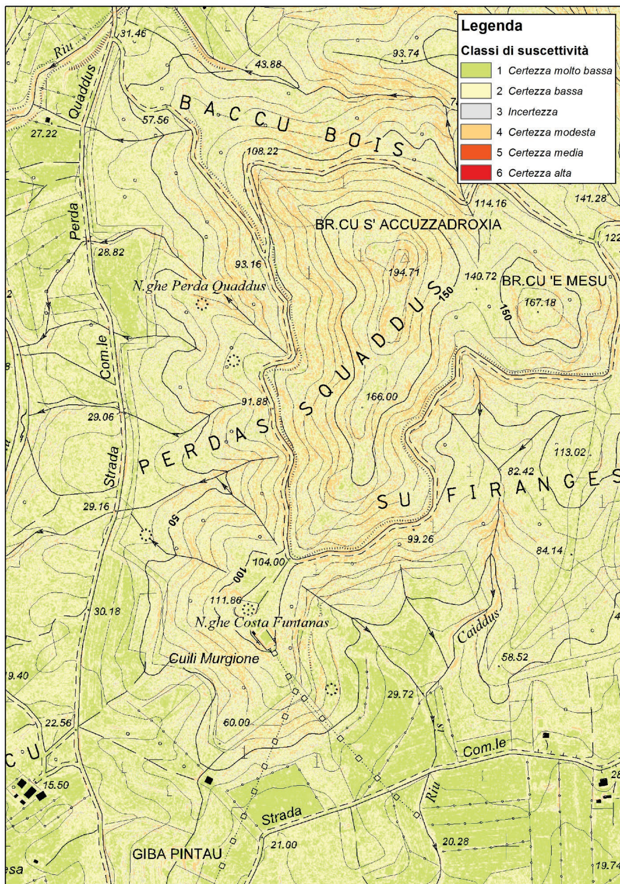
Figura 21 - Carta della suscettività da frana realizzata mediante la metodologia del CF
