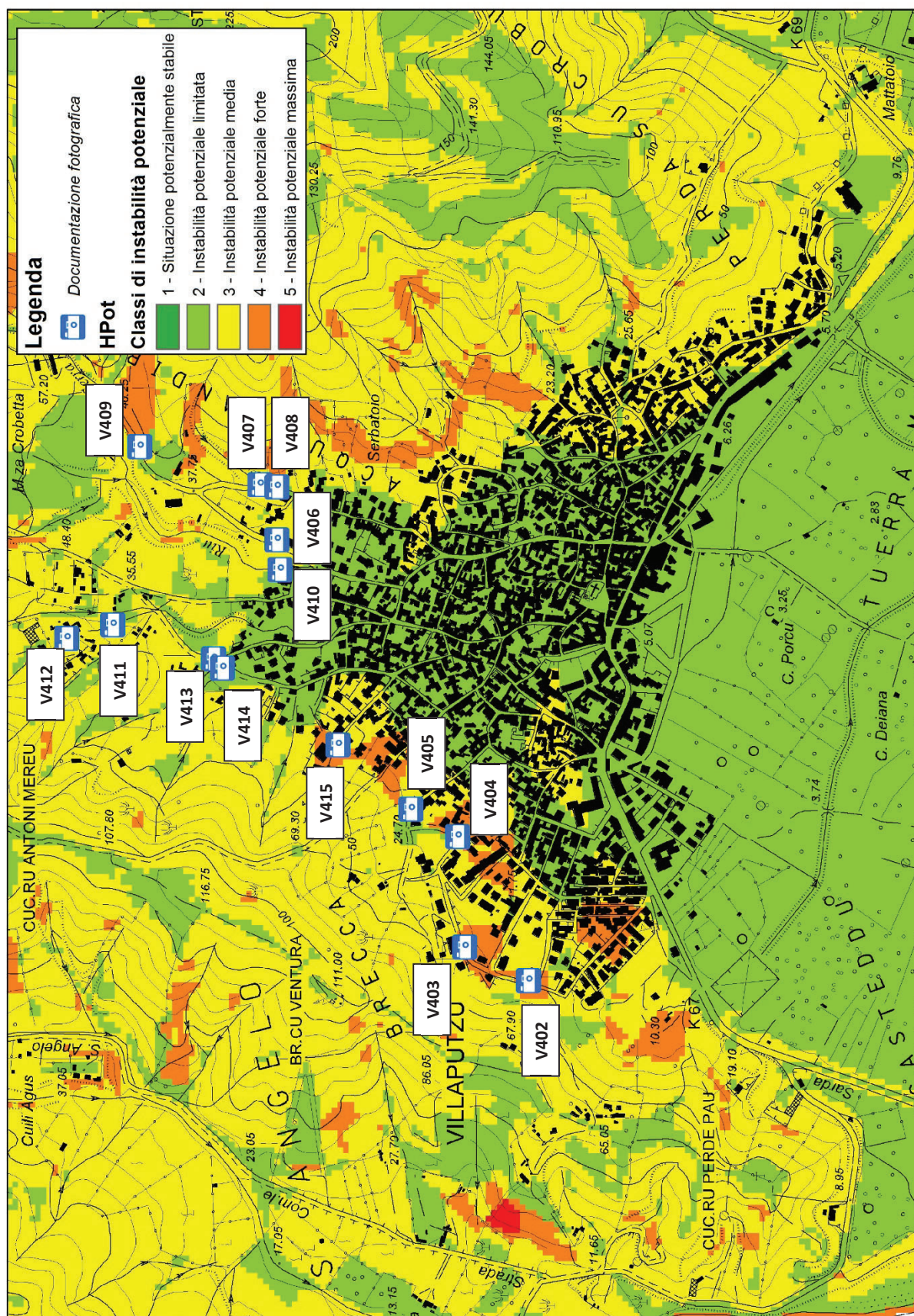
Figura 1 - Carta dell'instabilità potenziale redatta secondo le linee guida del PAI con ubicazione di alcuni scatti fotografici riportati nel testo.
