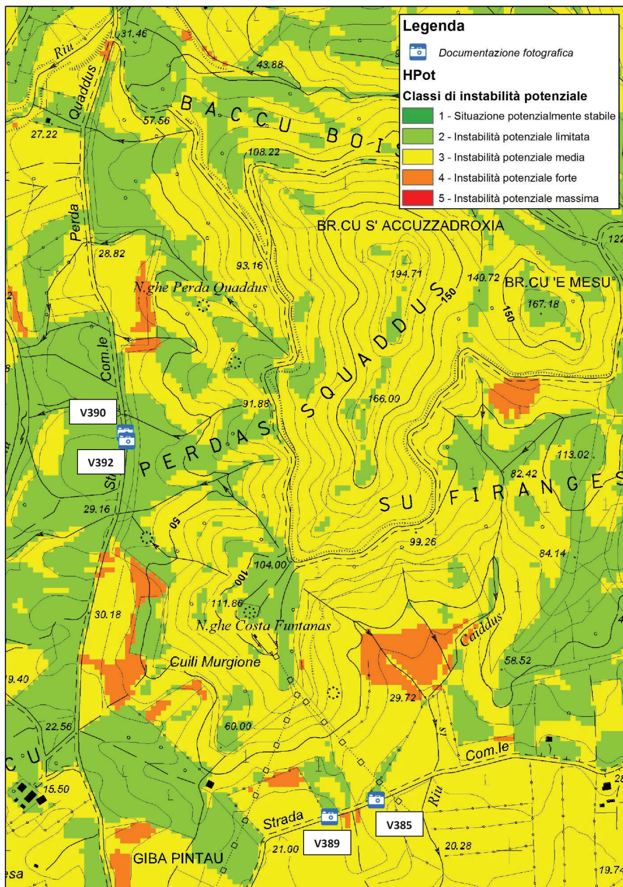
Figura 16 – Carta di instabilità potenziale per il settore di Perda Quaddus
